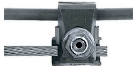
TND (Transtactor Nu Derivation) відгалуження «голим» проводом від СИП
