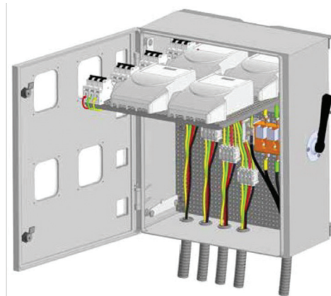
Обслуговування Шафи – доступність до вузлів та комплектуючих приладів
