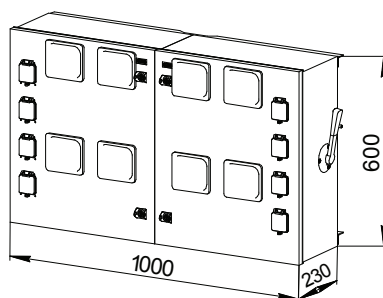
ARED-65-M8 Г Виконання: Г – горизонтальне
