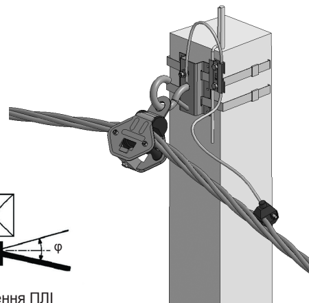
Кут відхилення ПЛІ
