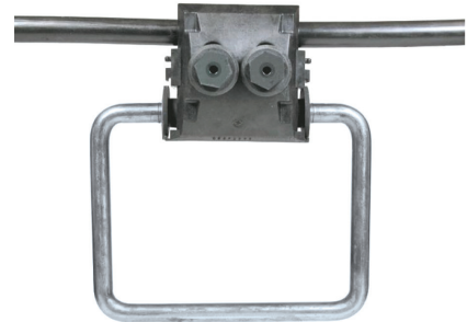
TND 28401 FA BI 95
