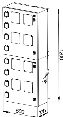
ARED-65-M8 В Виконання: В – вертикальне
